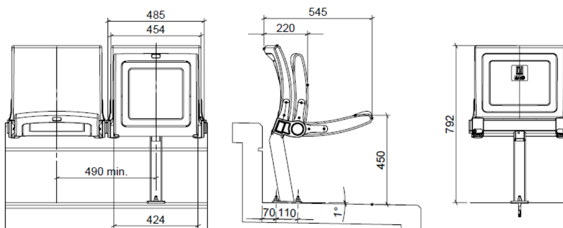
Rysunek 4.1: Podstawowe wymiary krzesła ARC LITE SLIM
